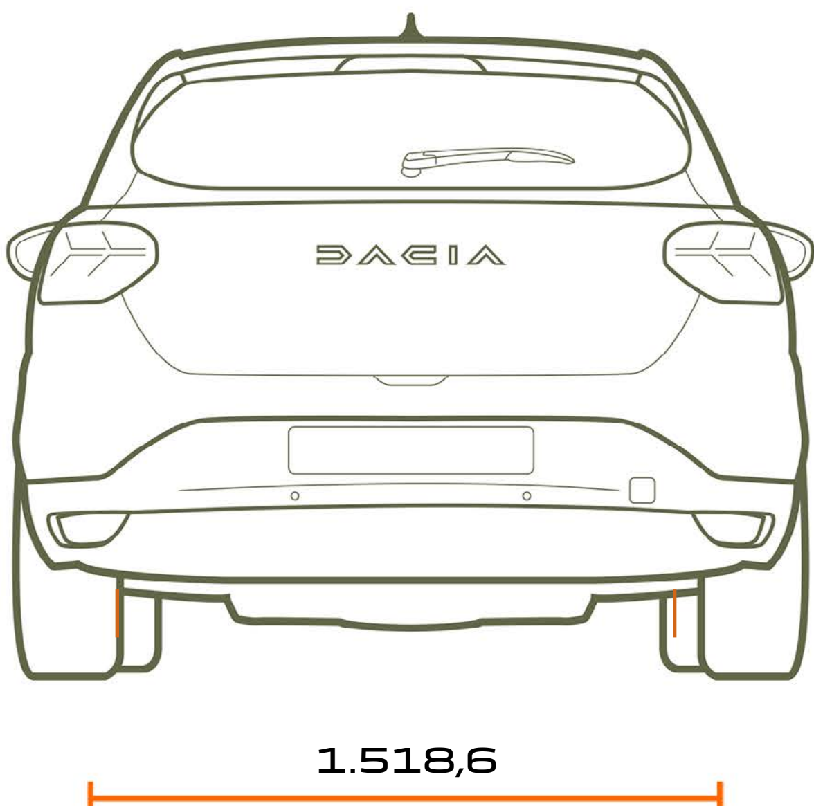
ACHTERAANZICHT
