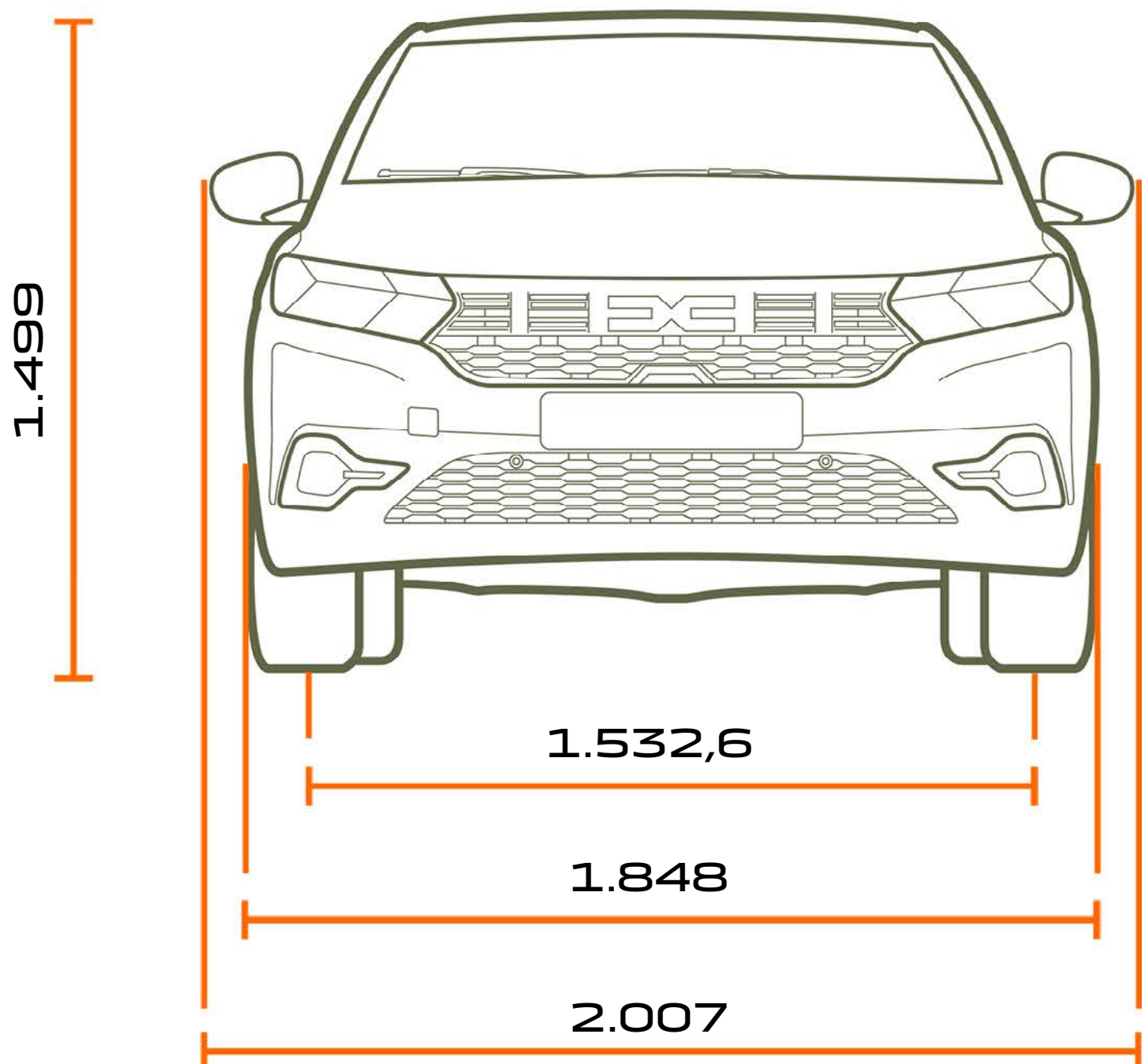
VOORAANZICHT
