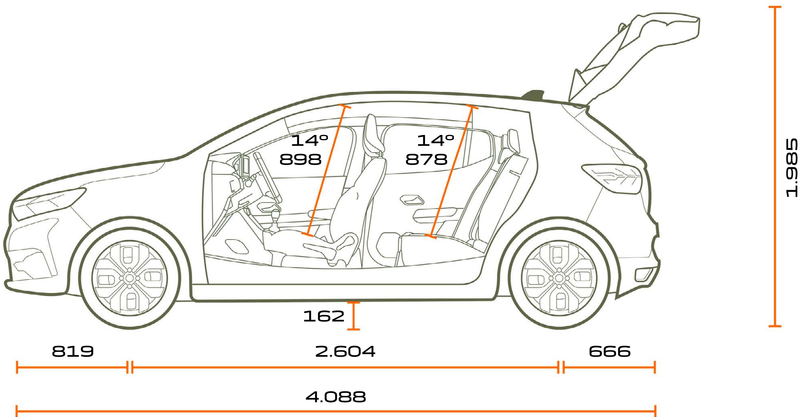
ZIJAANZICHT
