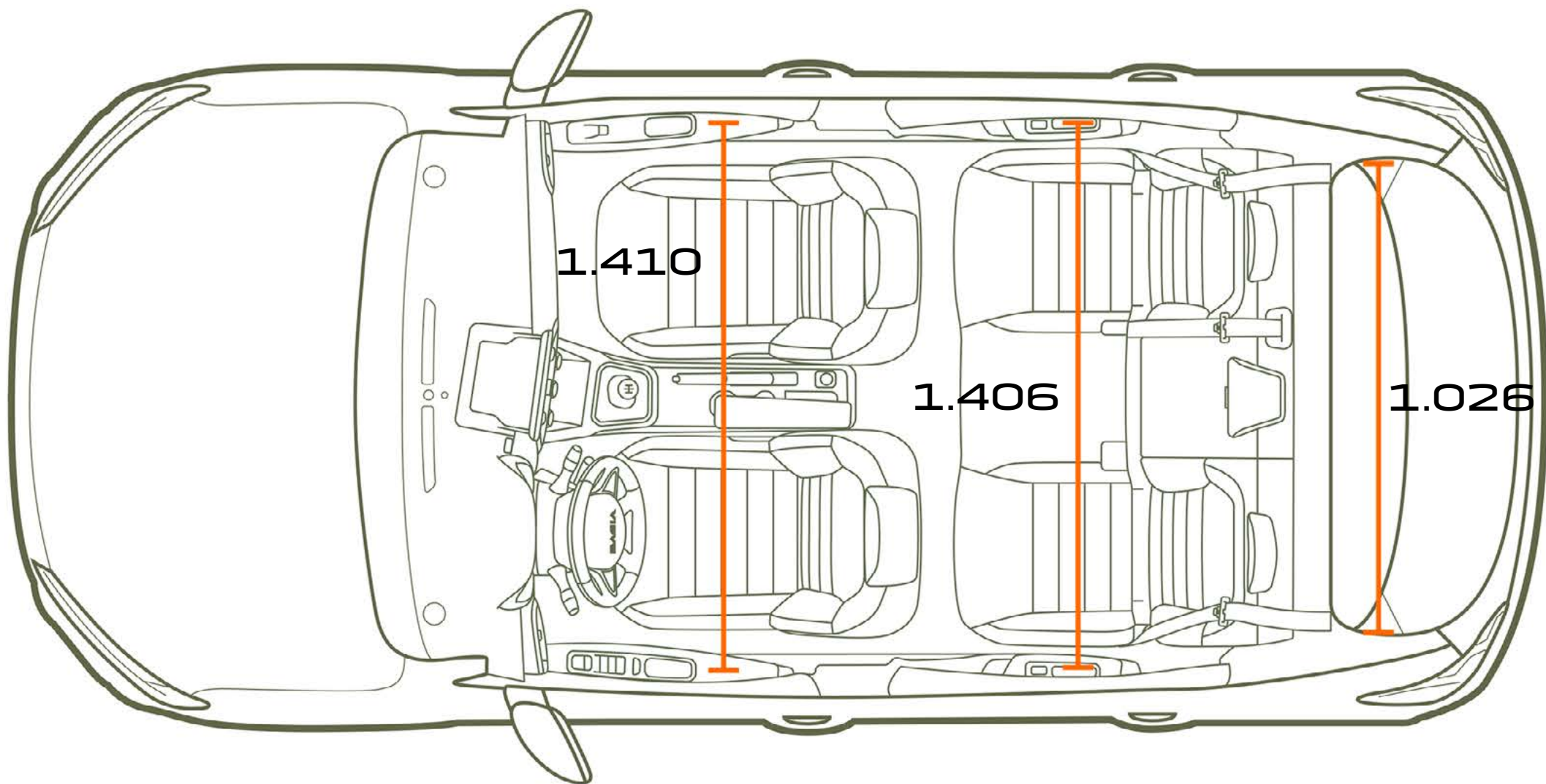
BOVENAANZICHT
